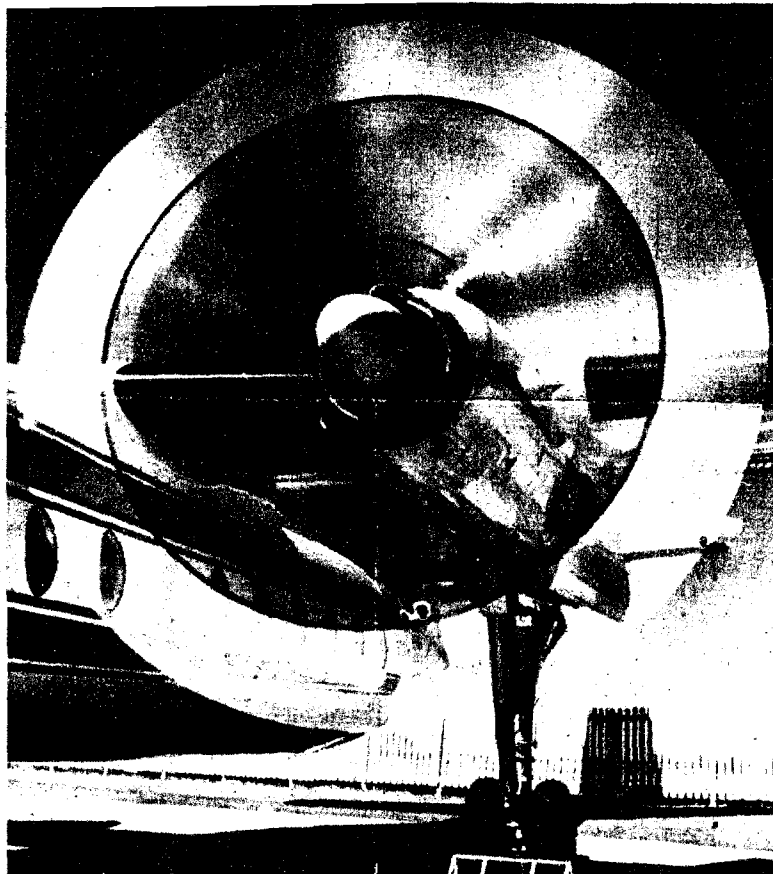
PROPULSOR DE UN AEROPLANO A REACCION.—Uno de los dos motores "Rolls-Royce", con que está equipado el aeroplano a reacción "Fairchild F-27", hace girar, a 1.300 revoluciones por minuto, a las cuatro hélices de este propulsor, que, revestidas con pintura "contra choques", parecen formar un disco transparente. (Foto Cifra.)
